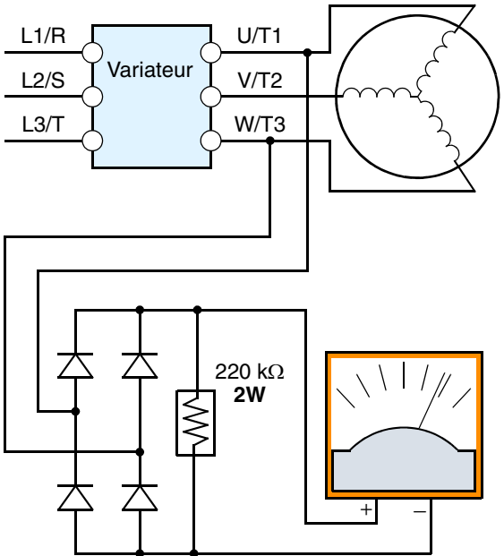
Mesure de tension en charge
