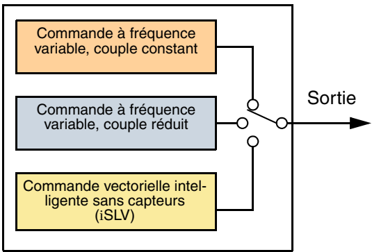
Algorithmes de commande du variateur
