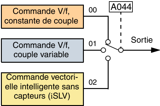
Algorithmes de commande de couple du variateur
