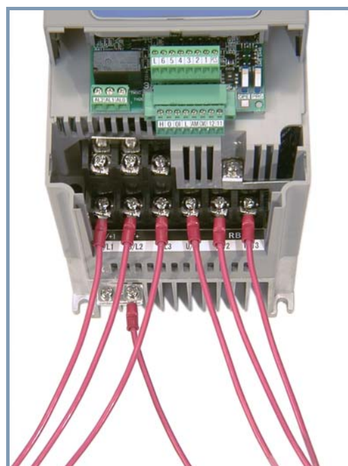
Exemple de câblage SJ200-037HFE/LFU
